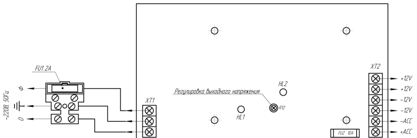
Рис. 1 Схема подключения
